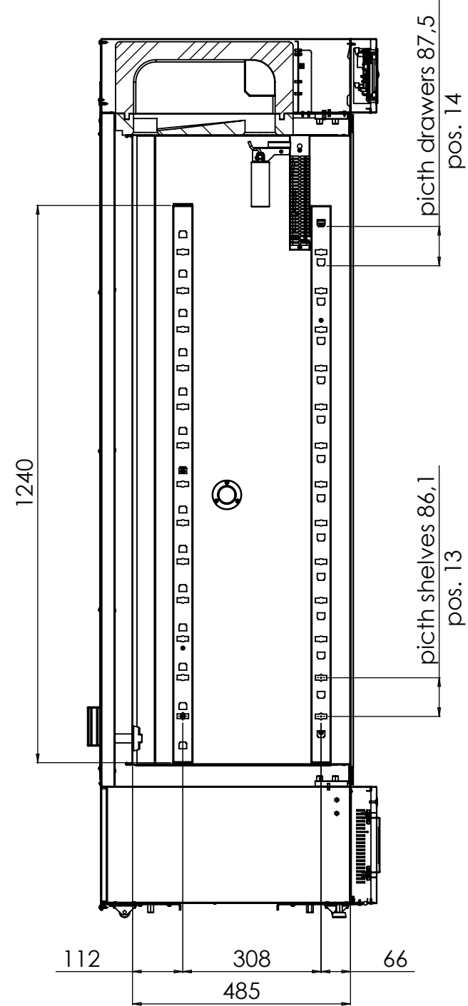
SECTION A-A
