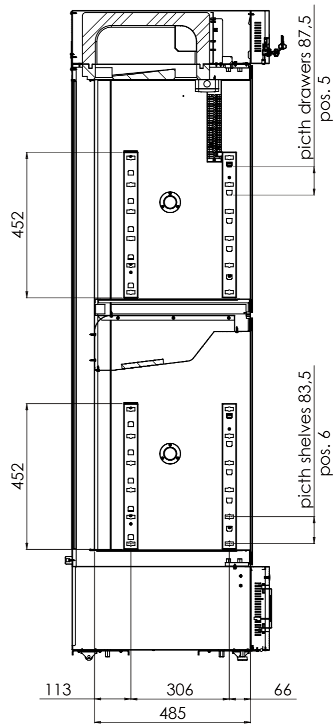
SECTION A-A
